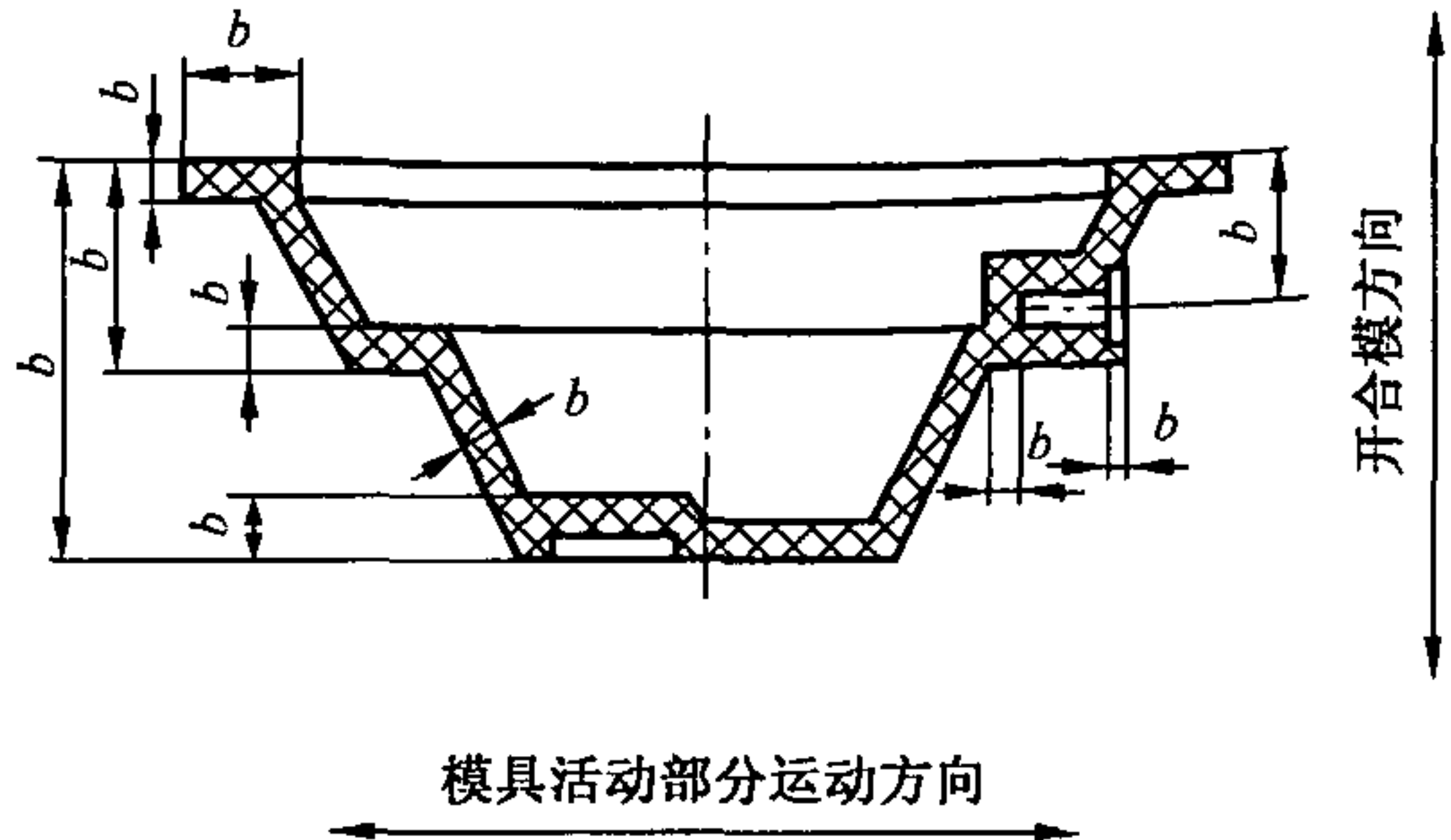
图 2 受模具活动部分影响的尺寸 b
