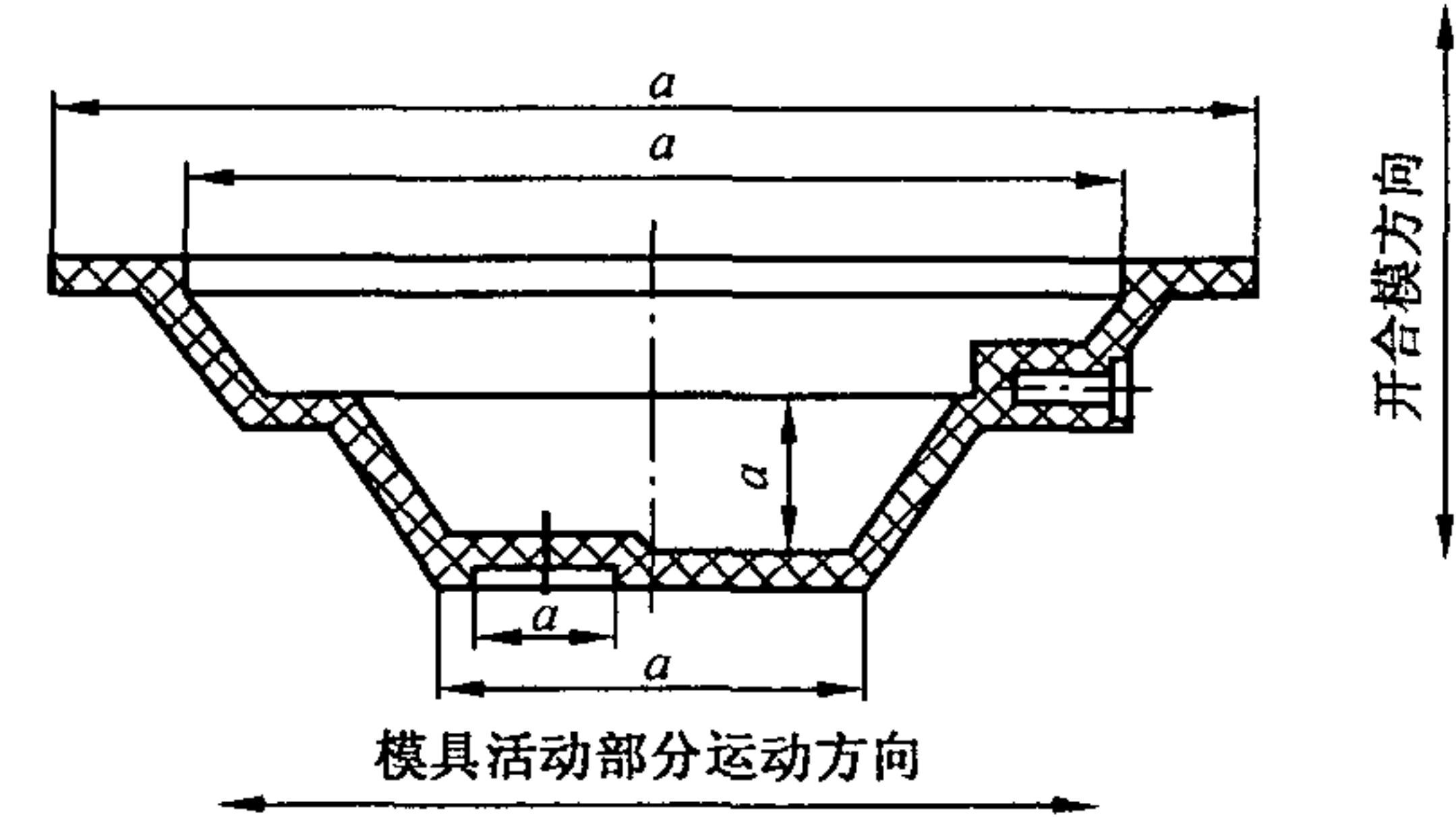
图 1 不受模具活动部分影响的尺寸 a
