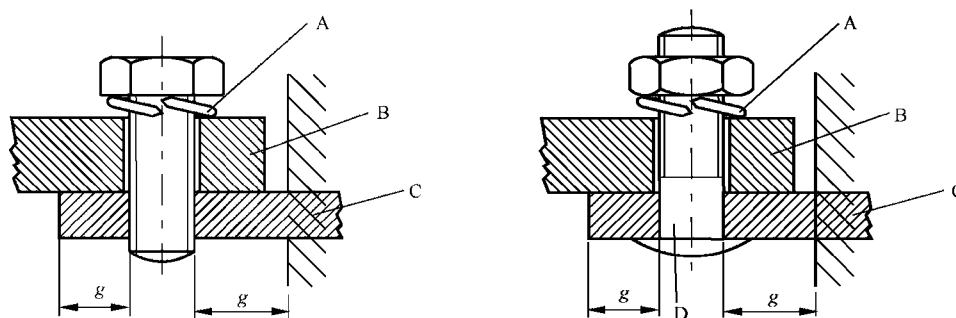
图 F.3 鞍形接线端子示例
