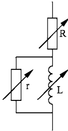
图 5 阻抗 Z 和 Z_1 的接线图
