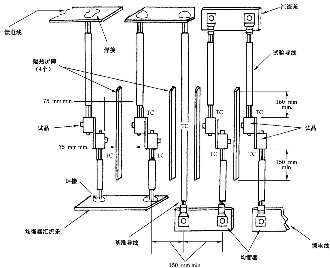
图 L.1 试验的总体布置
