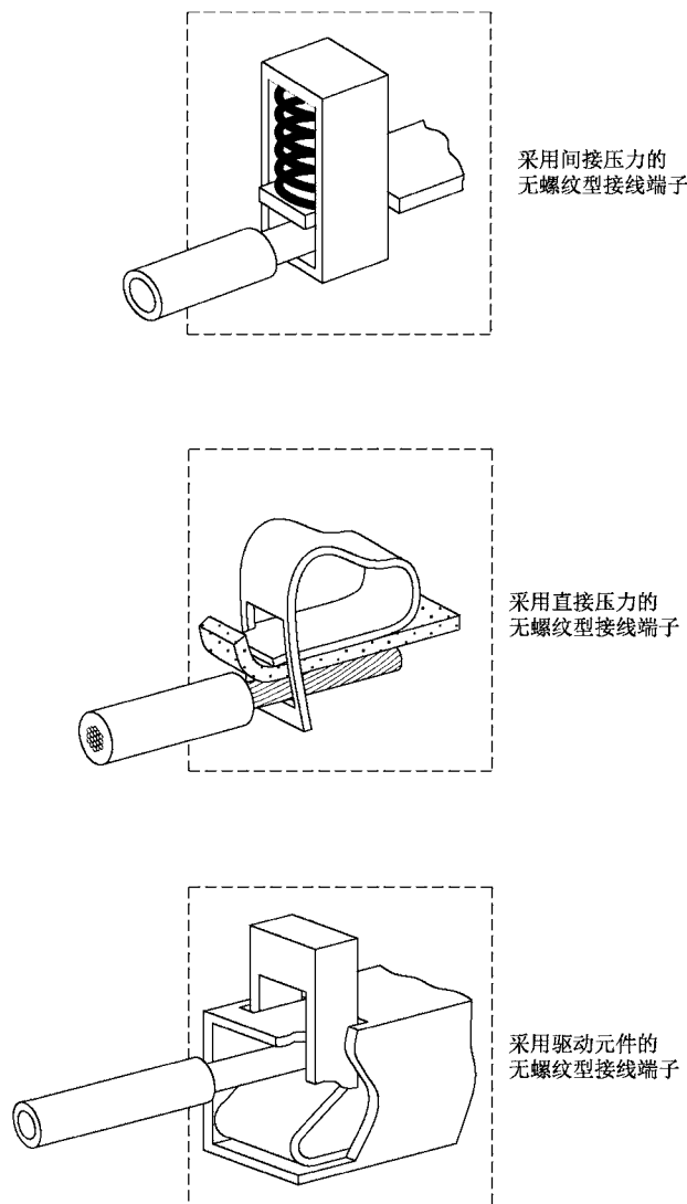
图 J.2 无螺纹型接线端子
