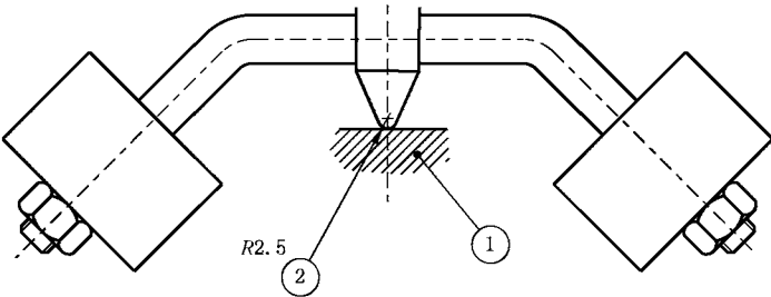
图 14 轨道安装断路器机械试验施加的力(9.13.2.4)
