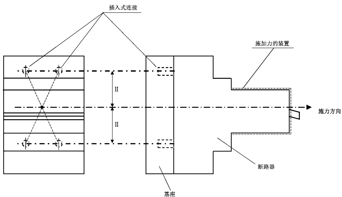
图 16 位置保持只与其插入连接有关的二极插入式断路器,机械试验施加力的示例(9.13.2.5)
