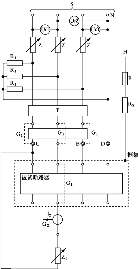
图 4 9.12.11.2.2 短路试验的典型电路图
