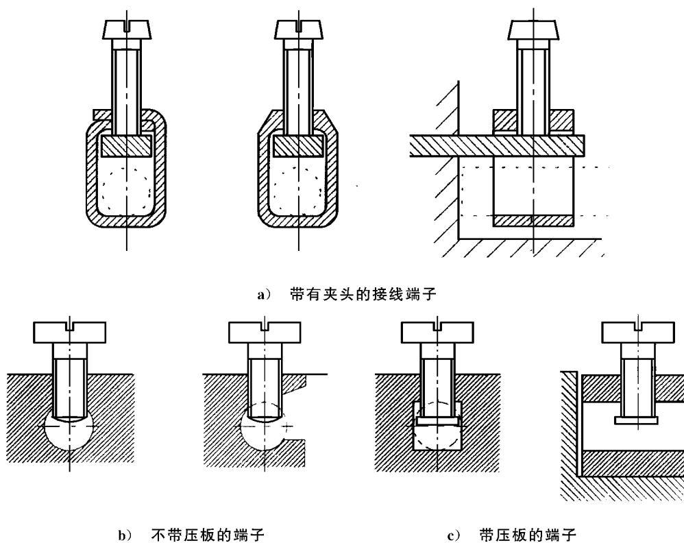
图 F.1 柱式接线端子示例
