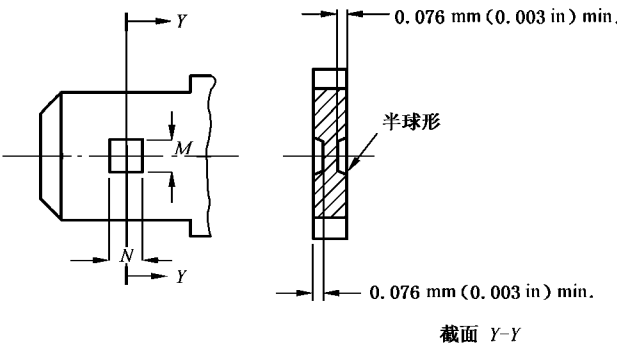
图 K.3 圆形凹痕定位扣的尺寸(见图 K.2)
