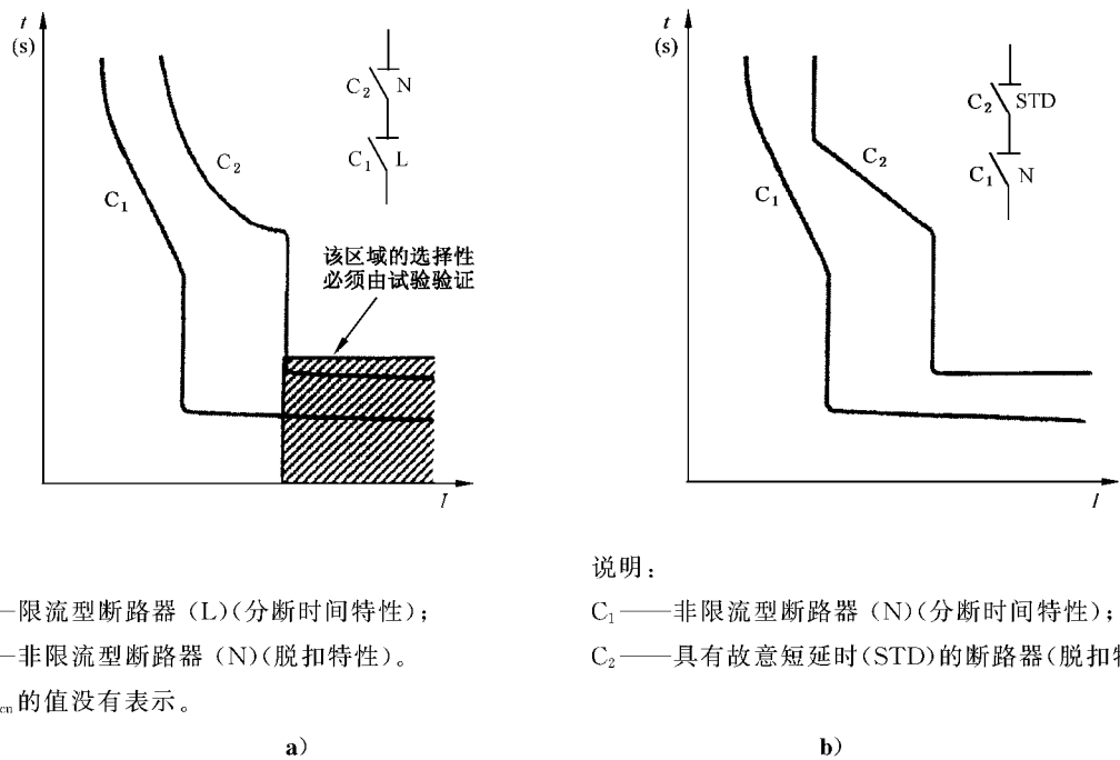
图 D.2 两个断路器之间的全选择
