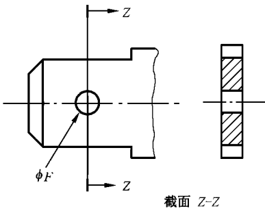
图 K.4 矩形凹痕定位扣的尺寸(见图 K.2)
