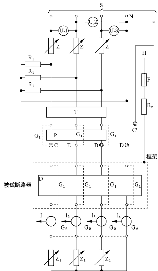
图 3 9.12.11.2.2 以外所有短路试验的典型电路图
