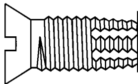
图 1 螺纹挤压成形自攻螺钉(3.3.13.1)
