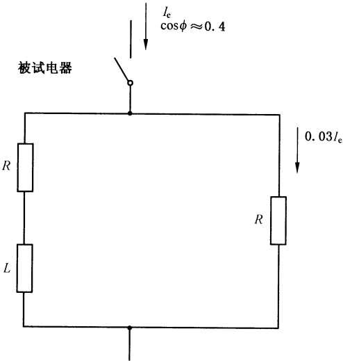
图 C.2 简化电路(见 C.3.2.2)
