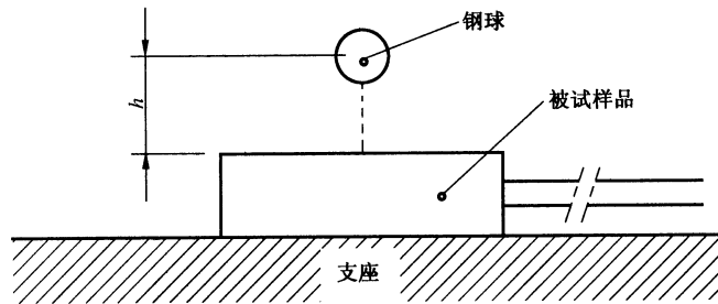
图 F.2 试验器具
