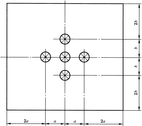
图 J.2 温升试验示意图
