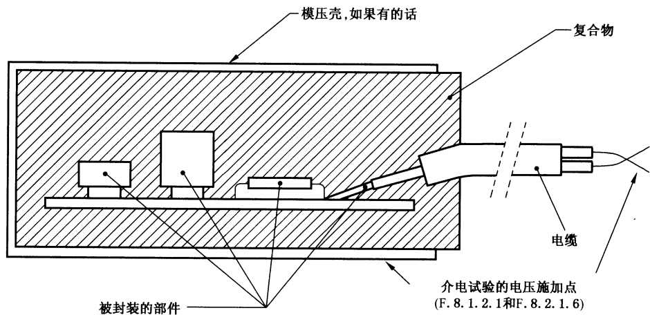
图 F.1 封装绝缘
