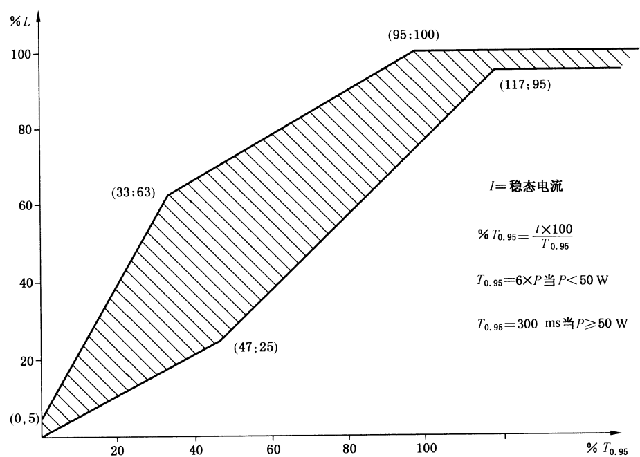
图 9 直流试验负载的电流/时间限值(见 8.3.3.5.3)
