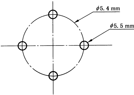
图 J.1 指示塔座的安装尺寸
