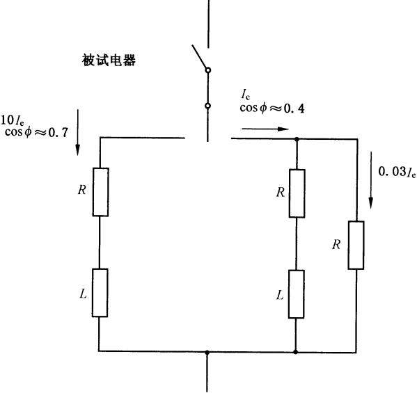
图 C.1 标准电路(见 C.3.2.2)
