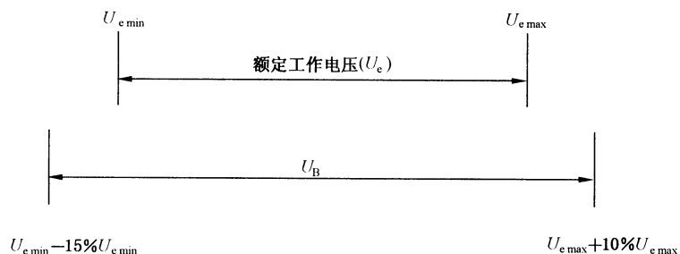
图 H.1 U_e 与 U_B 之间的关系
