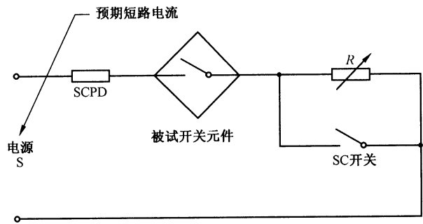
图 H.3 短路试验(见 H.8.6.1)
