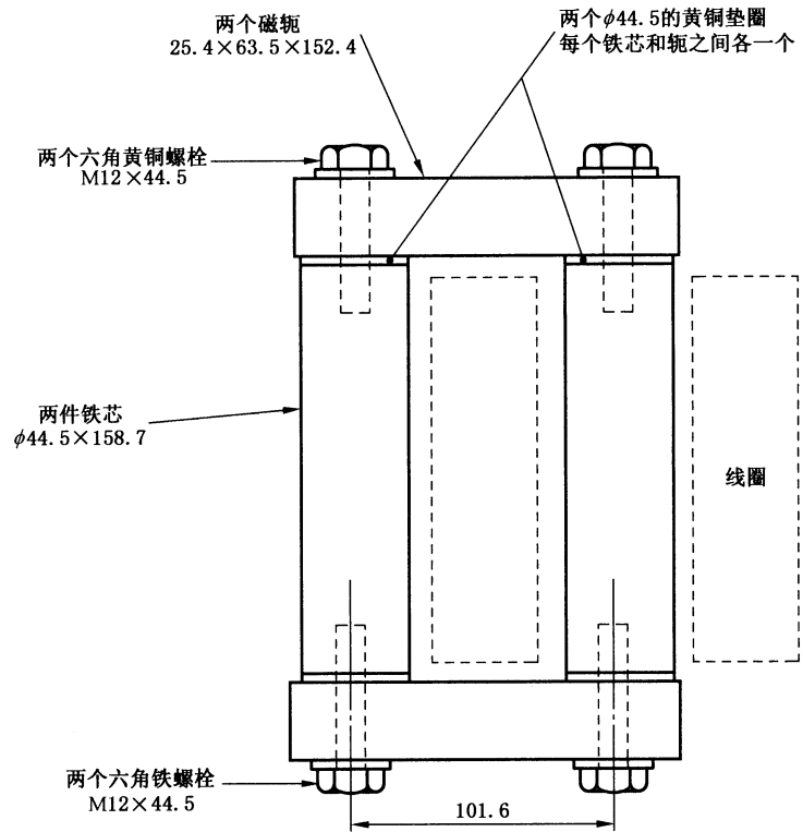
图 B.1 直流触头负载的结构尺寸
