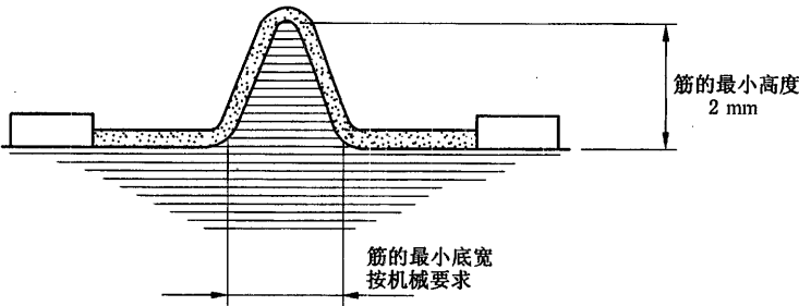
图 G.1 筋的测量
