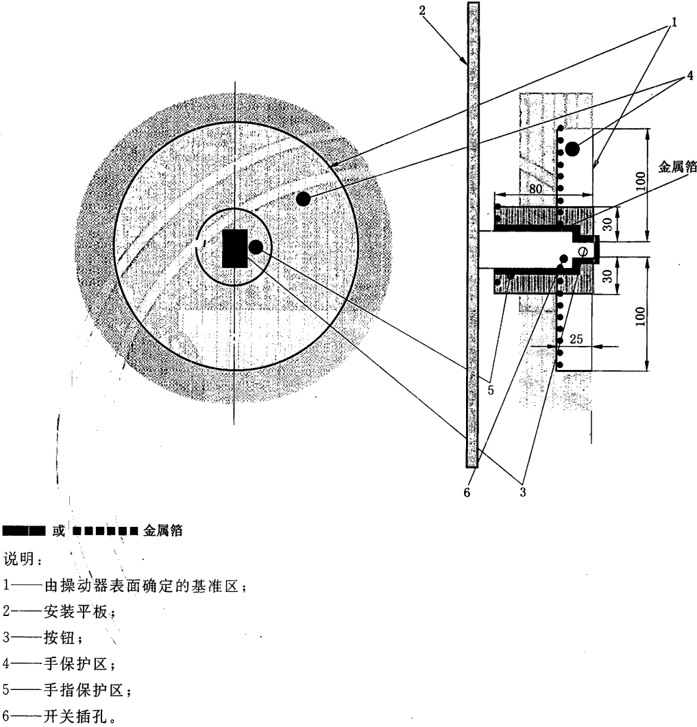
图 R.2 按钮操动的操作空间
