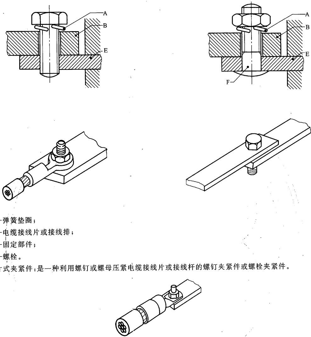
图 D.6 接线片式夹紧件
