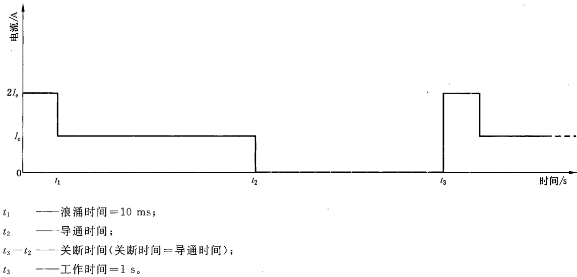
图 S.4 直流数字输出的暂时过载波形图
