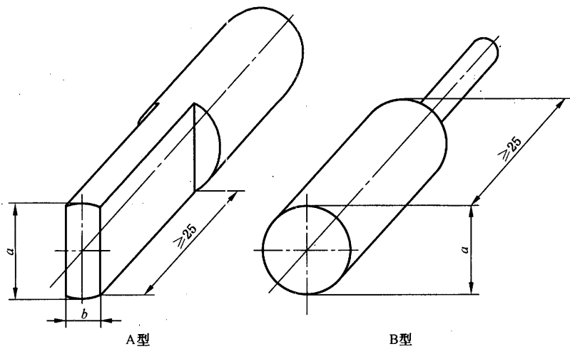
图 2 A 型和 B 型模拟量规 (见 8.2.4.5.2 和表 7)
