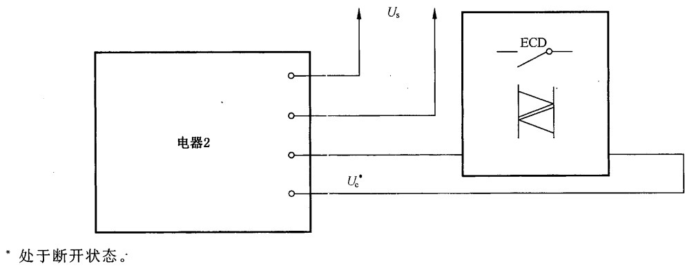
图 U.3 独立电源和控制输入
